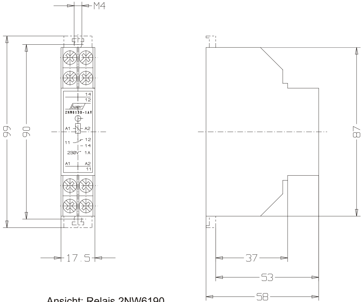
Ansicht: Relais 2NW6190
