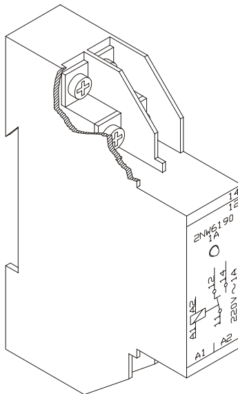
Ansicht: Relais 2NW6190
