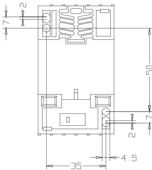
Ansicht Rückseite
