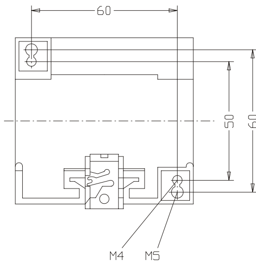
Ansicht: Relais 7PW0113-X
